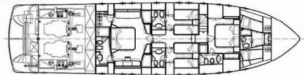
Ponte Sottocoperta / Lower Deck
